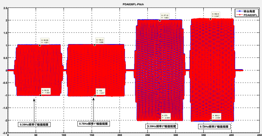
图 2 .pitch 方向摇摆数据, 分别为 0.39Hz 频率 1°幅值摇摆, 0.78Hz 频率 1°幅值摇摆, 0.39Hz 频率 2°幅值摇摆, 0.78Hz 频率 2°幅值摇摆。
