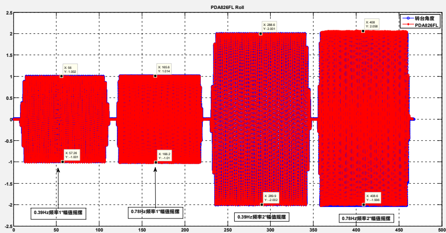
图 1 .roll 方向摇摆数据, 分别为 0.39Hz 频率 1°幅值摇摆, 0.78Hz 频率 1°幅值摇摆, 0.39Hz 频率 2°幅值摇摆, 0.78Hz 频率 2°幅值摇摆。
